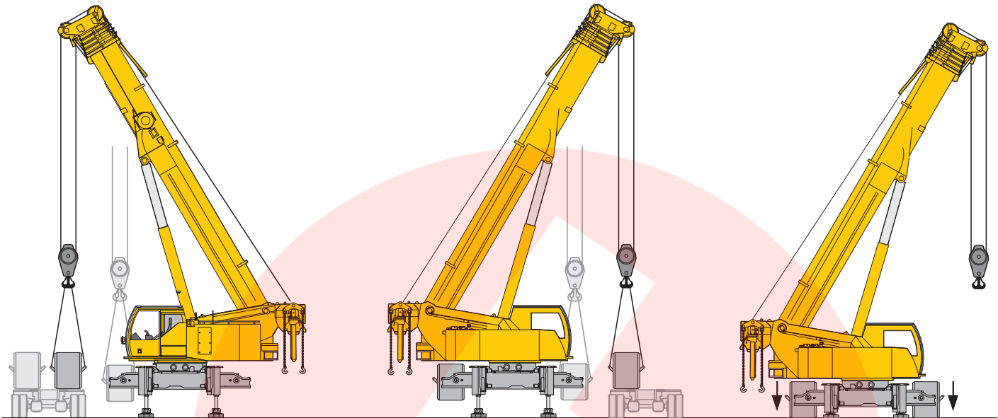
Montage der Raupen Crawler assembly Montage des chenilles Montaggio dei cingoli Ensamblaje de cadenas Монтаж гусениц
