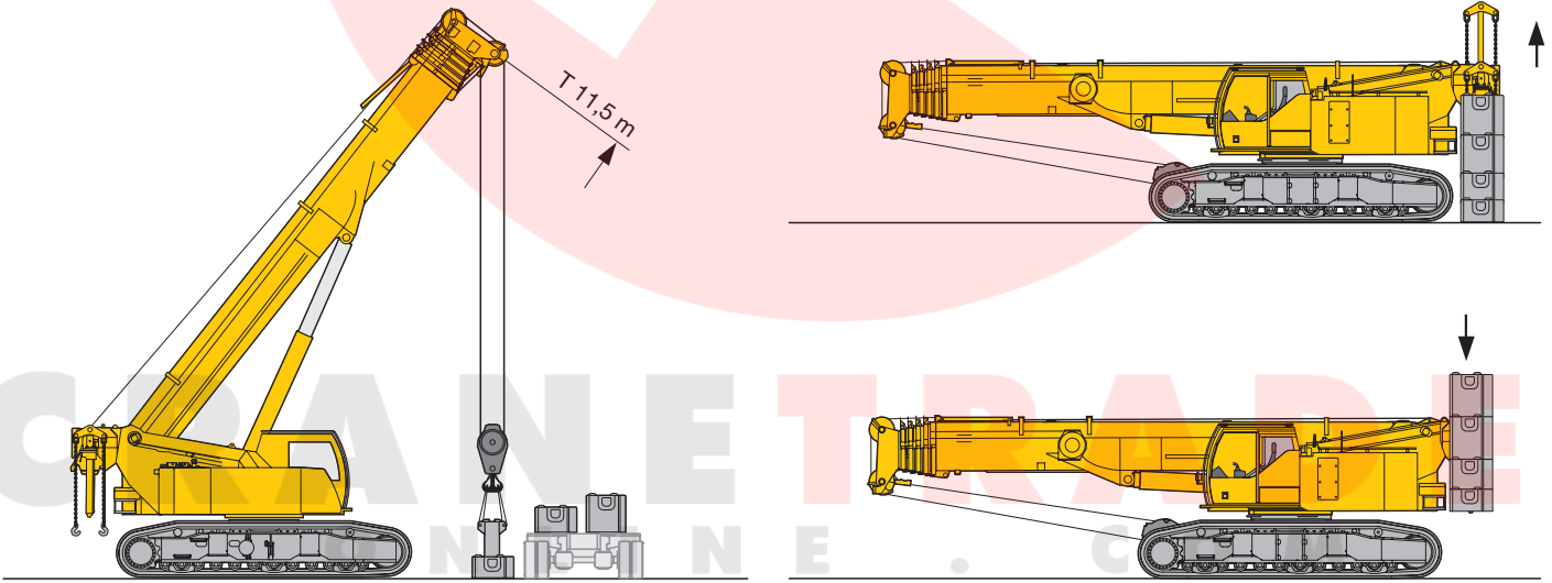
Montage Drehbühnenballast Assembly superstructure ballast Montage du contrepoids de la partie tournante Montaggio zavorra piattaforma girevole Montaje contrapeso superestructura Монтаж противовеса поворотной илатформы
